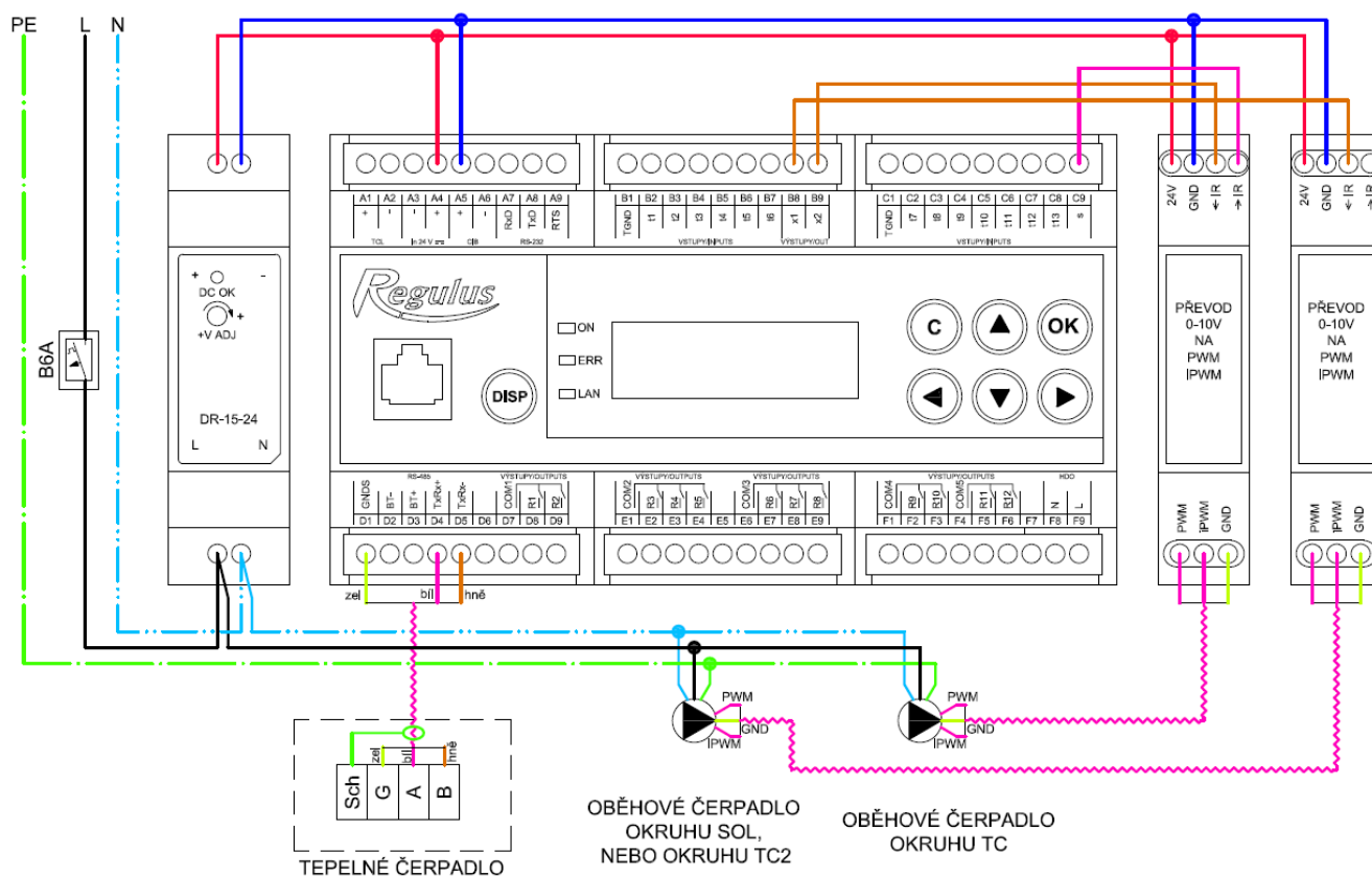
Obr. zapojení napájecího zdroje, modulu iPWM pro řízení oběhového čerpadla tepelného čerpadla, solárního oběhového čerpadla a tepelného čerpadla k regulátoru.
