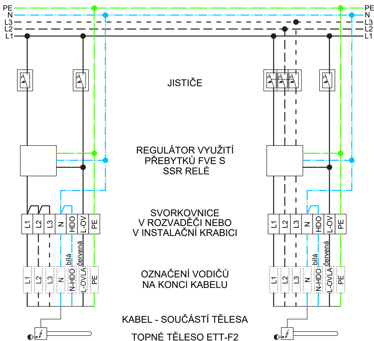
VARIANTA S JEDNOFÁZOVOU FVE
