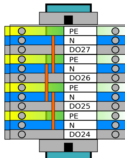
Pomocná svorkovnice nastavitelných výstupů
