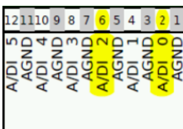
Svorkovnice pro připojení teplotních čidel
